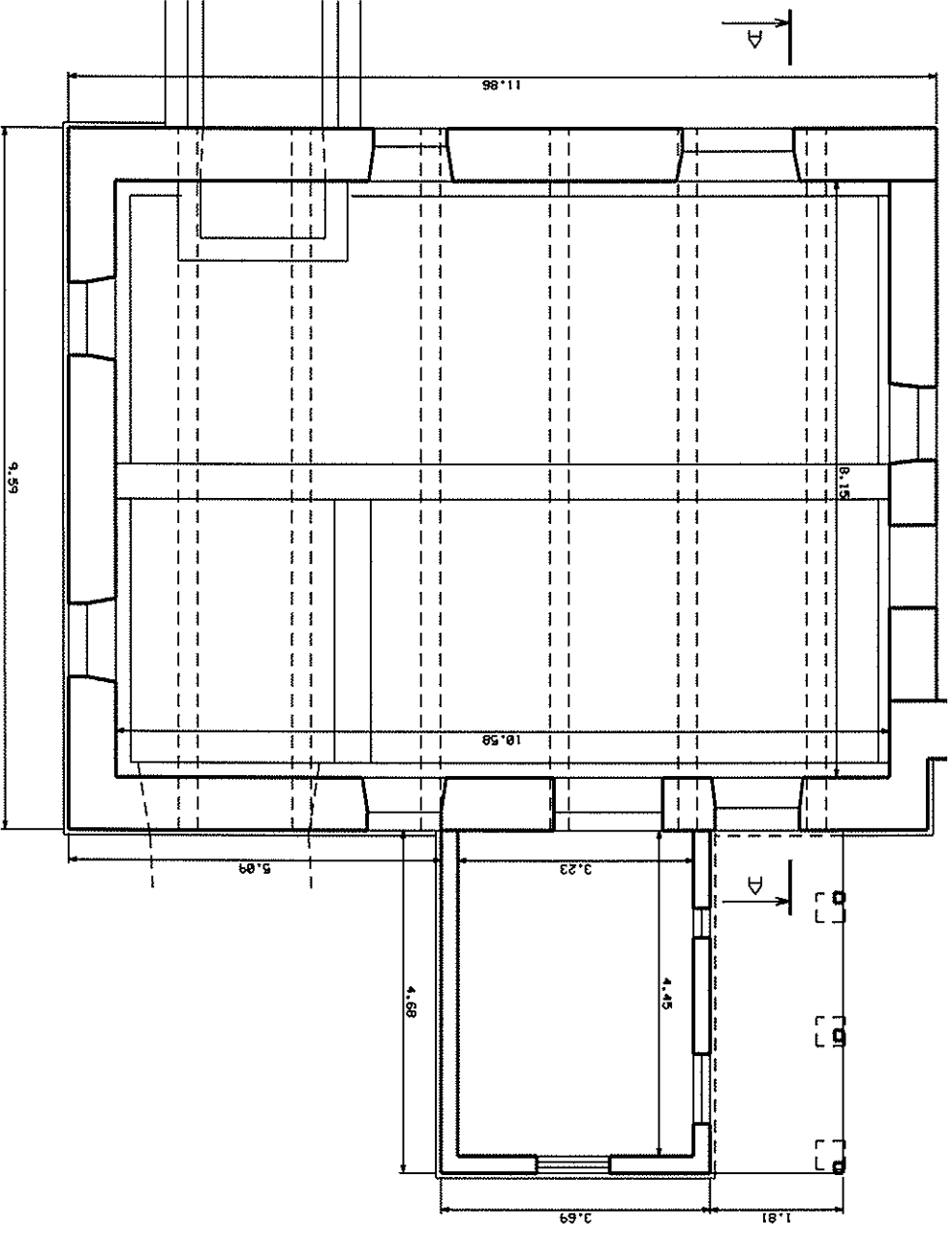
Põhiplaan
