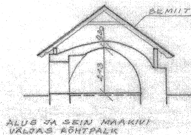
LÖIGE B-B
