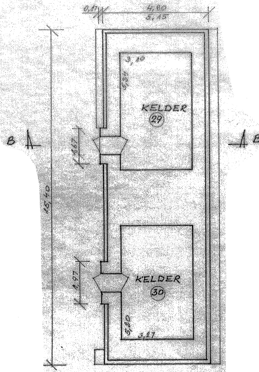
KELDER -2- PÕHIPLAAN
