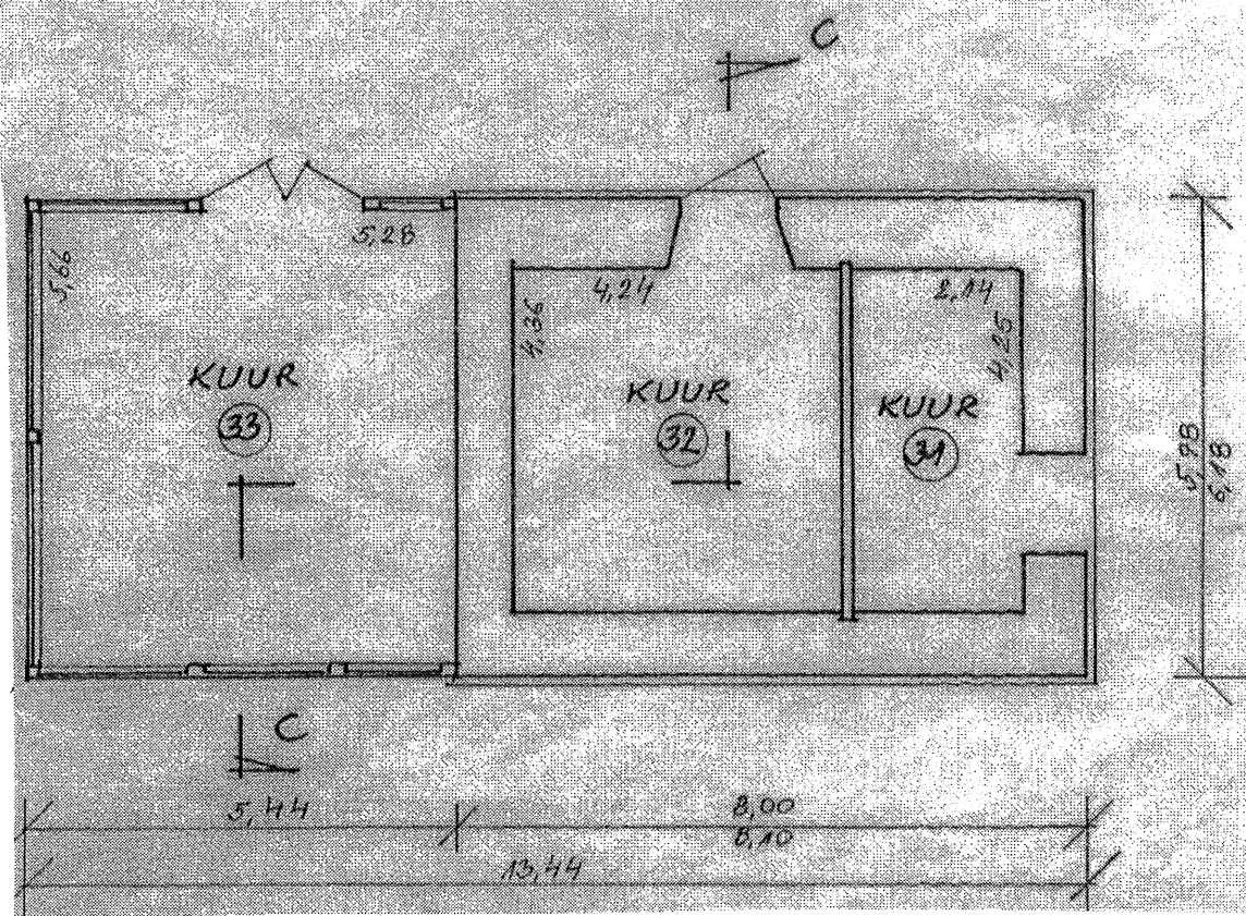
TÖÖRIISTAKUUR -3- PÕHIPLAAN
