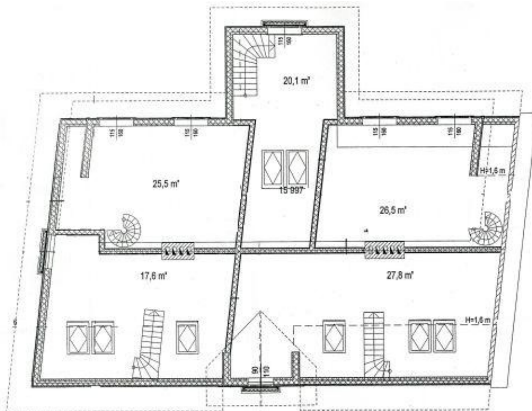
Katusekorruse ümberehituse plaan
