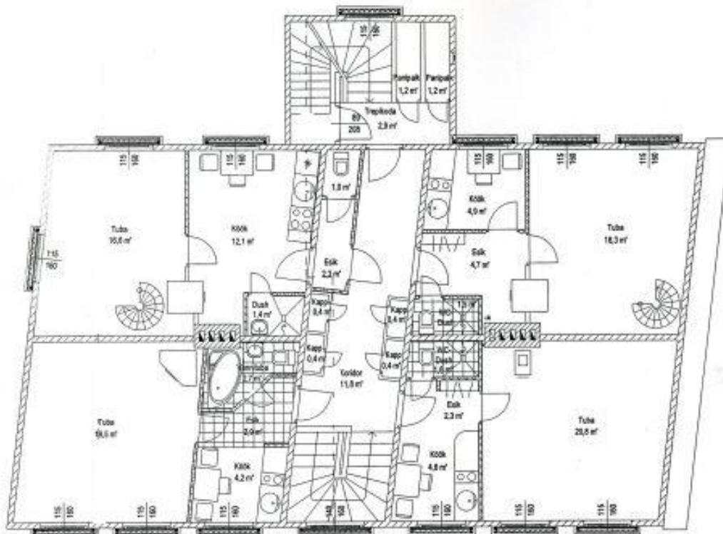
2 korruse ümberehituse plaan
