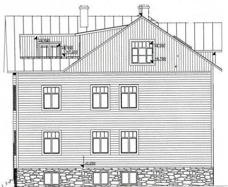
Otsavaade
