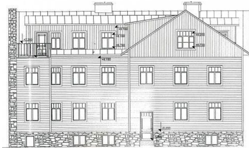
Tagantvaade
