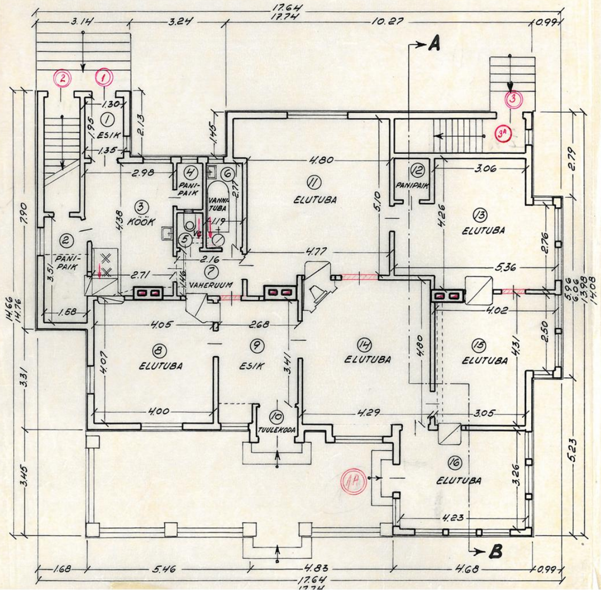
Lisa 9. Keldi ja esimese korruse plaan. Allikas: Tallinna Linnaarhiiv TLA.1396.6.1934
