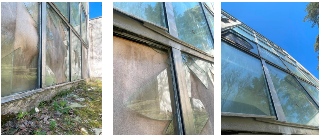
Ill 97, 98, 99. I korpuse kõige suurem aken läbi 4 korrust, metallist aknaraam
